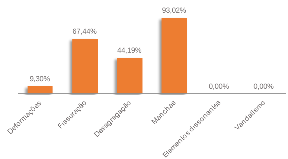
42 | Patologias ao nível da fachada
